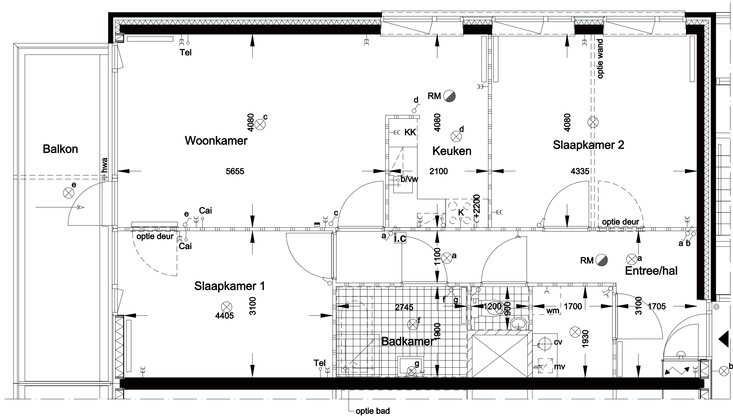
Verkooptekening type 02
